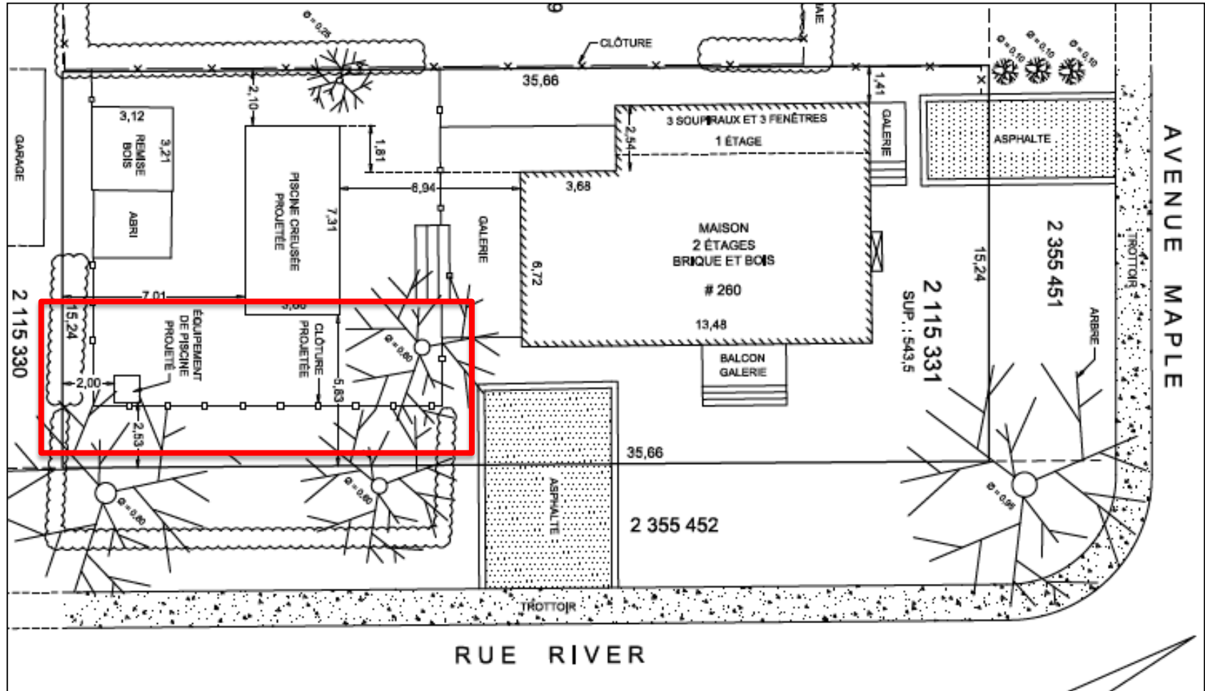
Plan d'implantation
